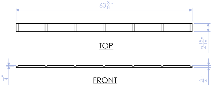
DELB-RB-11 BOTTOM CAP: LONG SIDE 3/4" PLY QTY:1
