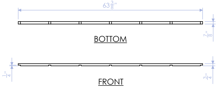
DELB-RB-7 TOP CAP: LONG SIDE 3/4" PLY QTY:1
