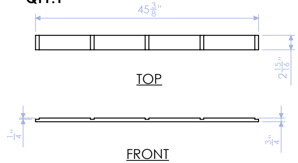
DELB-LB-11 BOTTOM CAP: LONG SIDE 3/4" PLY QTY:1
