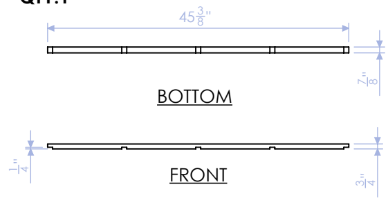
DELB-LB-7 TOP CAP: LONG SIDE 3/4" PLY QTY:1
