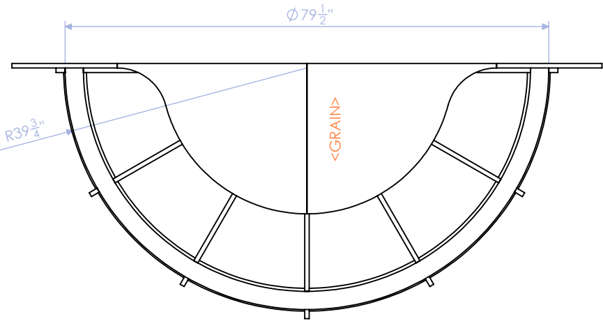
TOP
