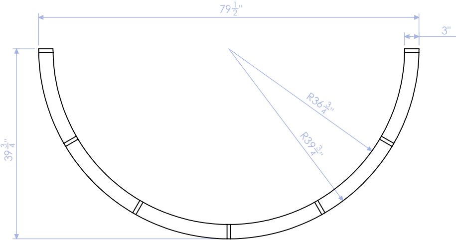
BOTTOM
