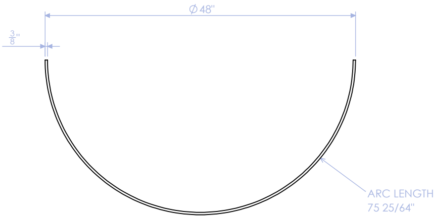
TOP
