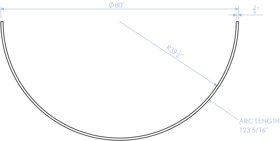
TOP
