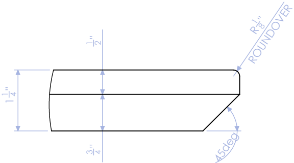
EDGE DETAIL AA
