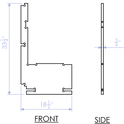
GPH-100-LF-5 BACK WRAP 3/4" KERF CORE QTY: 1
